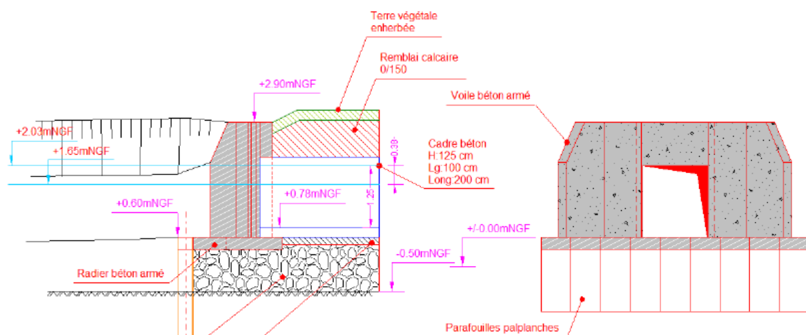
Figure 8 : Description de l'ouvrage de confortement des berges – Source : Présentation AVP
