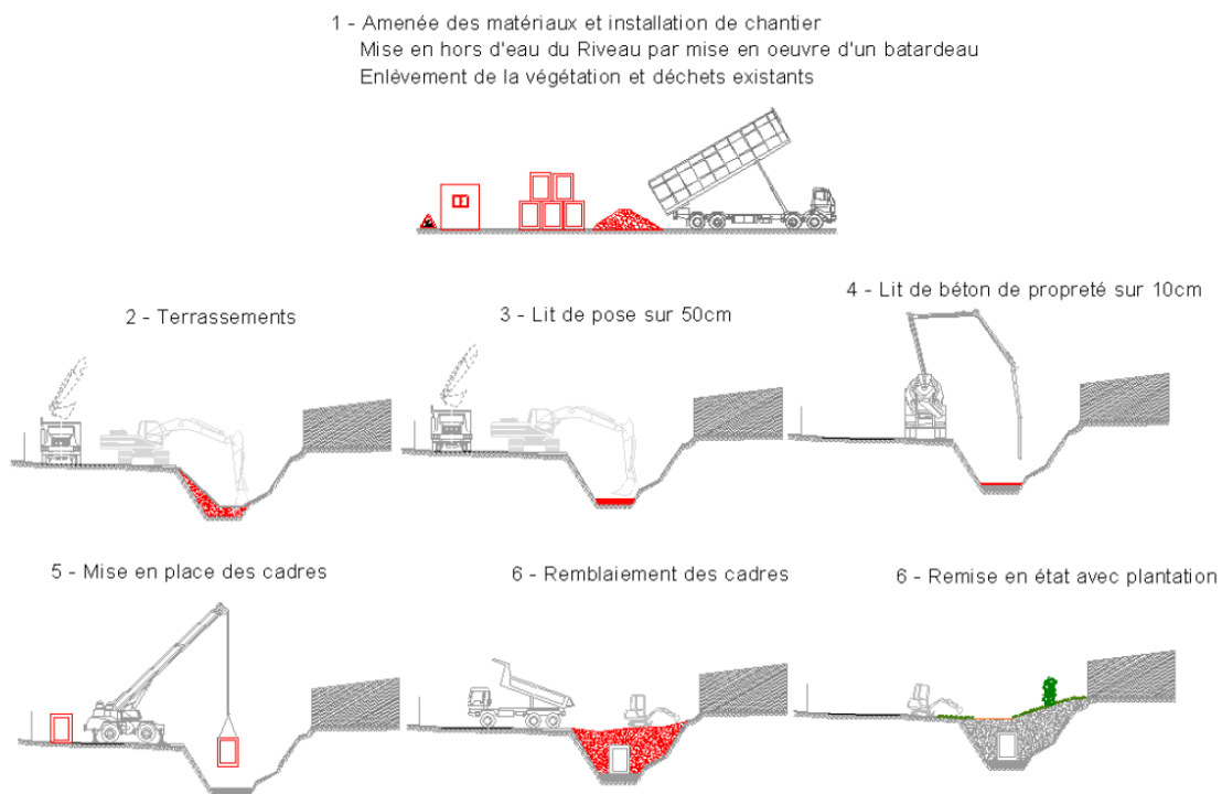
Figure 9 : Schématisation des travaux de confortement des berges – Source : Présentation AVP
