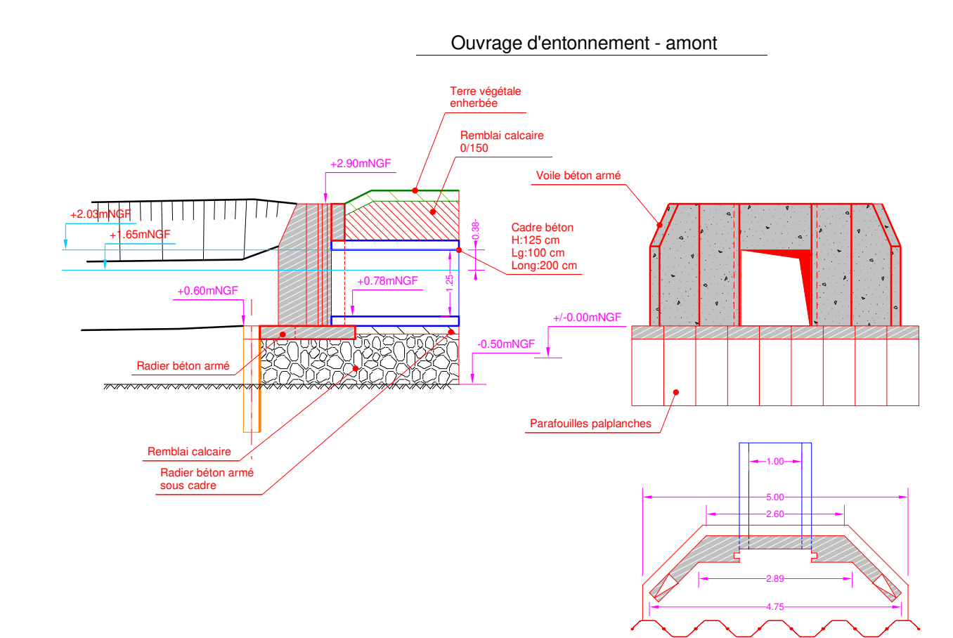
Détail sur ouvrage d'entonnement 1/100
