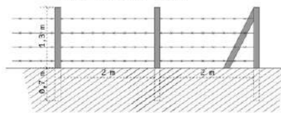
Figure 16 : Profil et exemple de clôture pâturage (Source : Etude paysagère PVIII)
