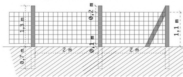
Figure 17 : Profil et exemple de clôture herbagère (Source : Etude paysagère PVIII)
