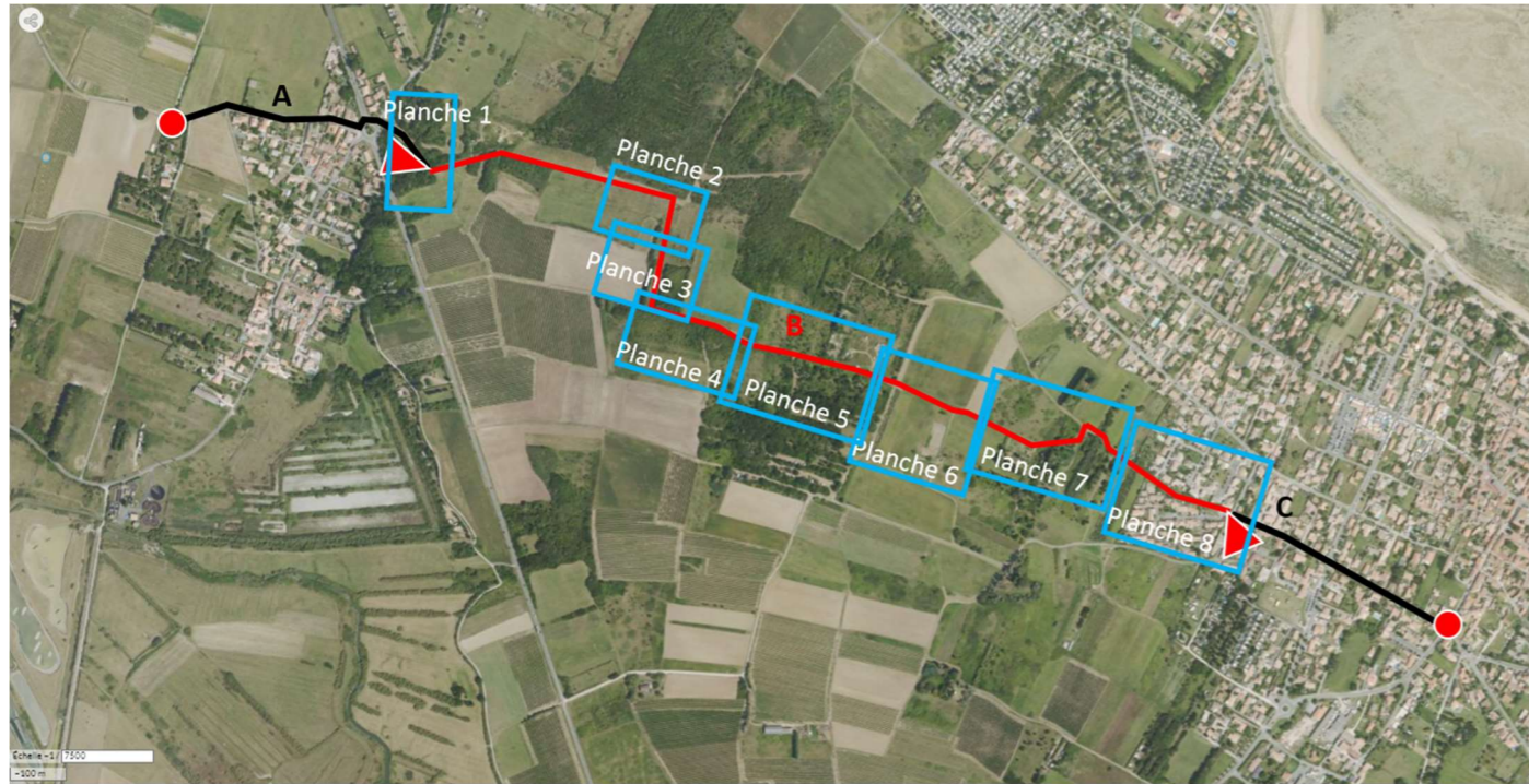
Figure 41 - Plan de situation des planches de plan topographique de l'état actuel du terrain (Source : CDCIO)
