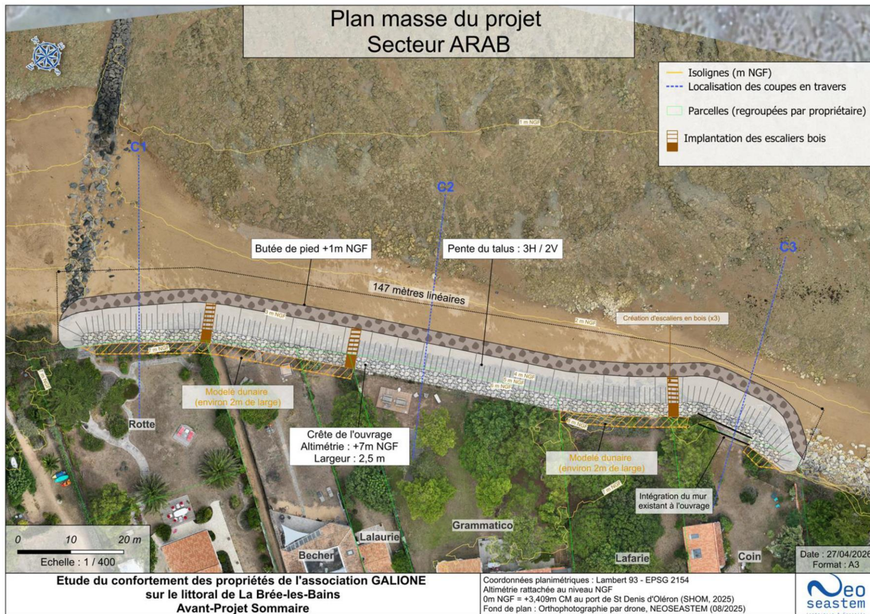
Planche 10 : Plan masse du secteur ARPPN (Neoseastem, 2026)
