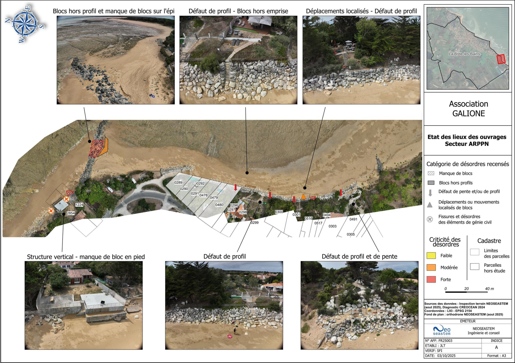
Planche 7 : Etat des lieux des ouvrages – Secteur ARPPN (Neoseastem, Etudes techniques préliminaires, 2025)
