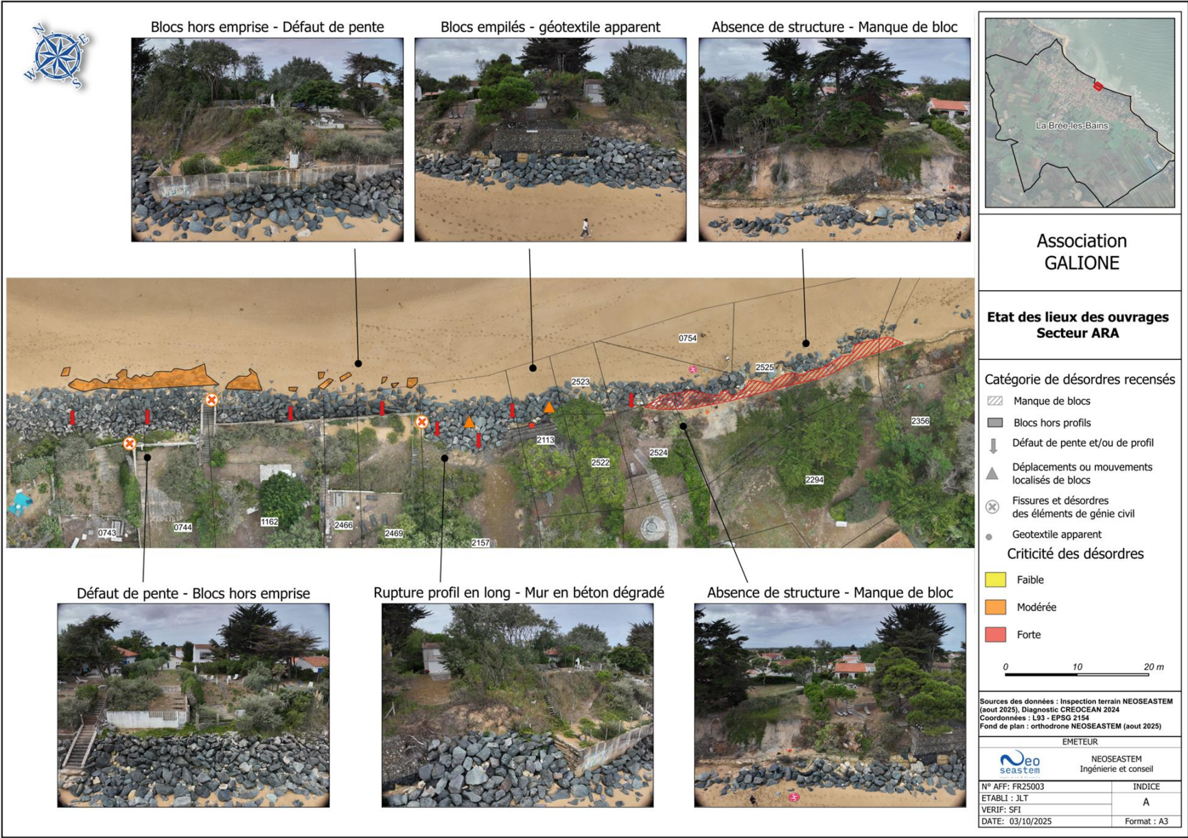
Planche 5 : Etat des lieux des ouvrages – Secteur ARA (Neoseastem, Etudes techniques préliminaires, 2025)
