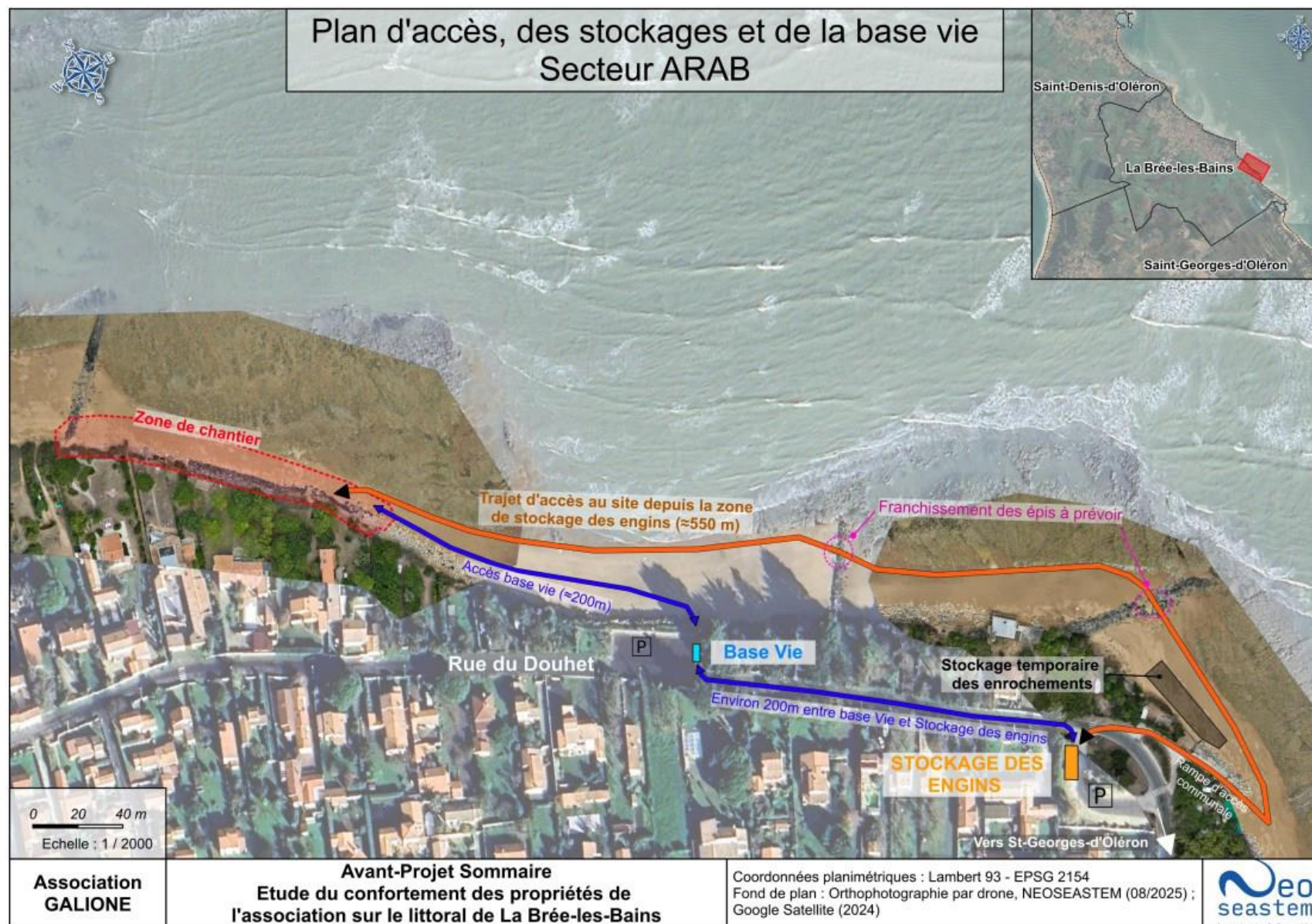
Planche 13 : Plan d'accès, zone de stockage et base vie – Secteur ARAB (Neoseastem, APS, 2026)
