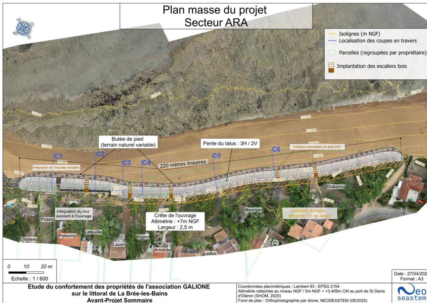
Planche 9 : Plan masse du secteur ARAB (Neoseastem, APS, 2026)
